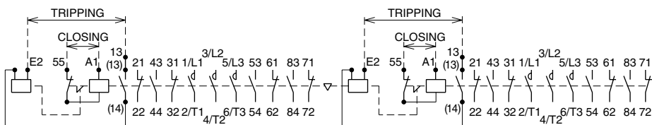
SL(D)-2xN600, N800
