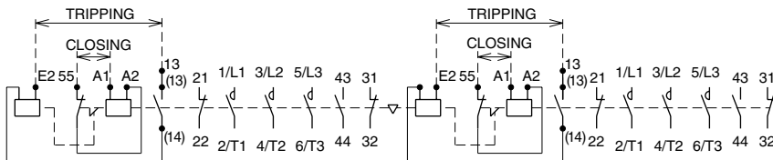
SL(D)-2xN80~N400
