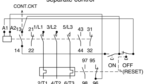
MS-N50~N95PM
