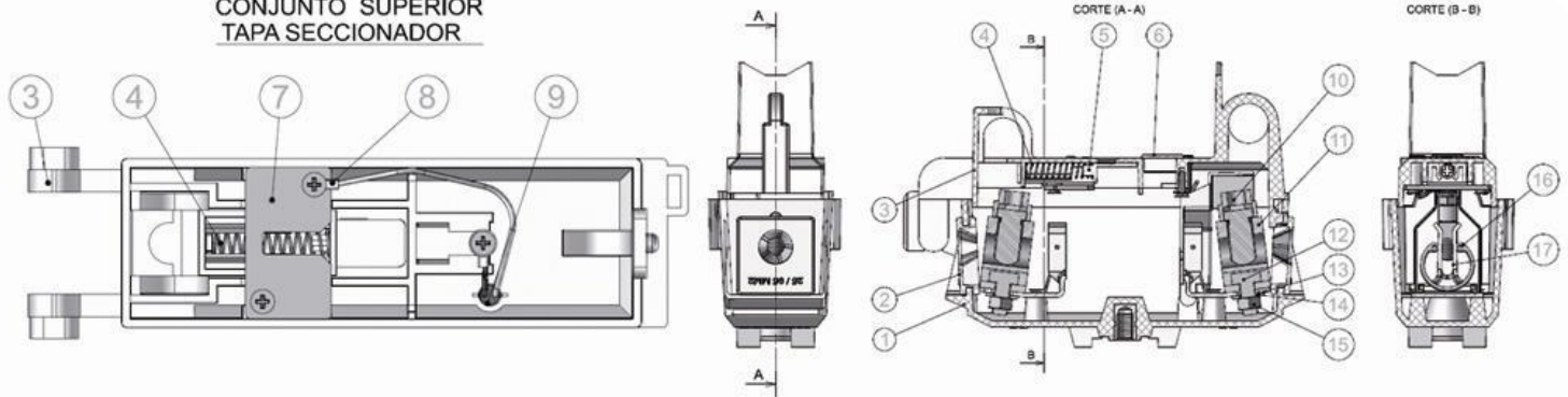
CONJUNTO INFERIOR CUERPO SECCIONADOR
